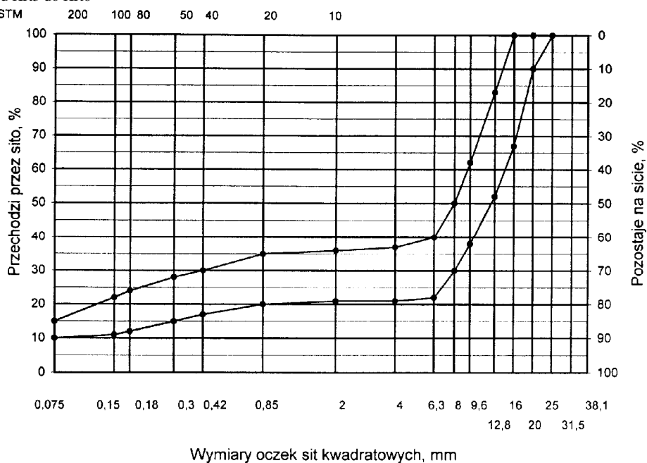
Rys. 5. Krzywe graniczne uziarnienia mieszanki mineralnej BA od 0 do 20 mm (mieszanka o nieciągłym uziarnieniu) do warstwy ściernalnej nawierzchni drogi o obciążeniu ruchem od KR3 do KR6
